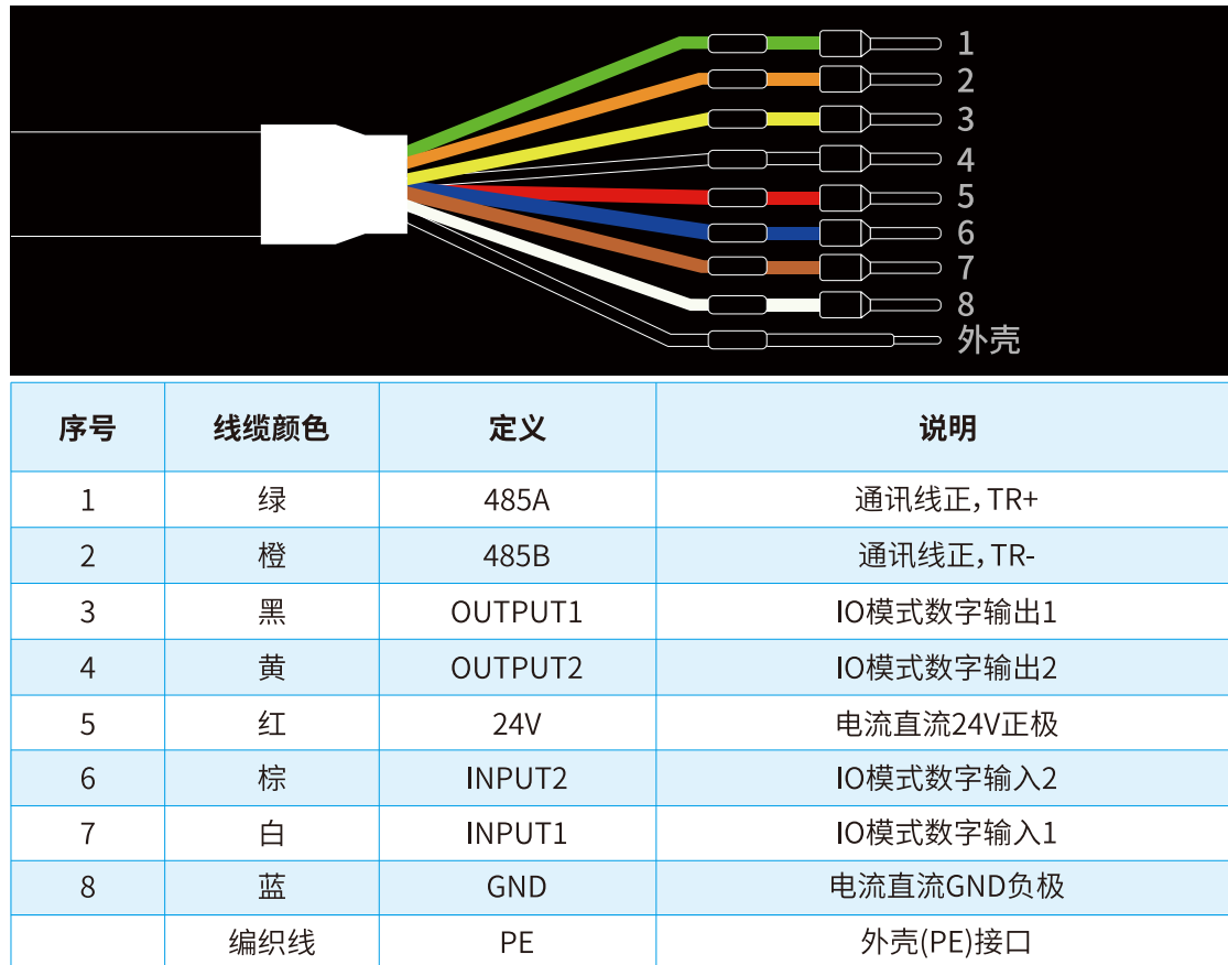
图1.1 线缆线标图
