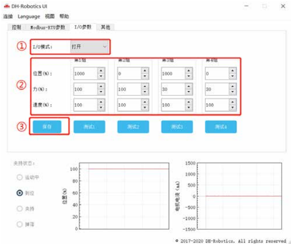
图2.5 (b) 打开IO模式
