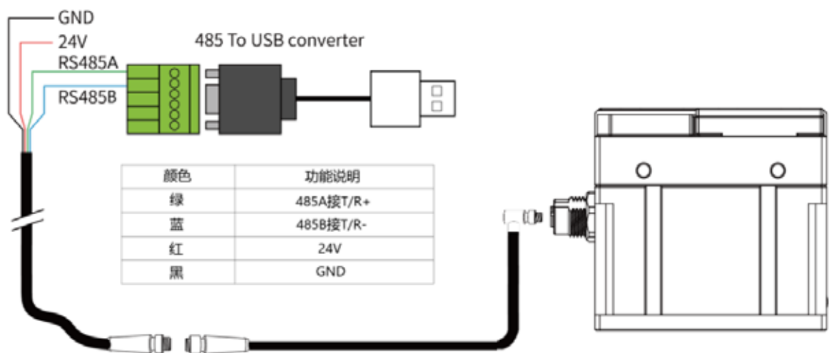
图2.1 RS485连接方式图 (此图为蓝色线标接线图, 黄色线标参考表1.3接线即可)
